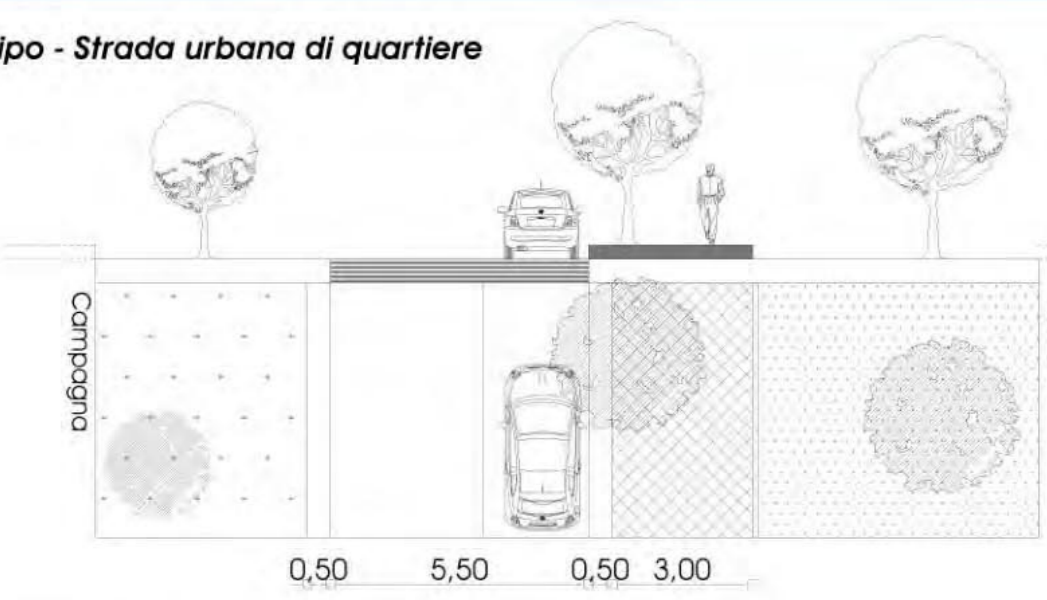
Sezione tipo - Strada locale urbana pubblica
