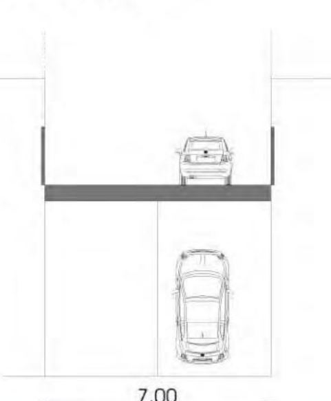
Sezione tipo - Strada locale urbana privata
